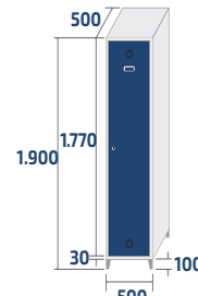
SV-50/1 COD: 45001 28kg · 0,48m 3
