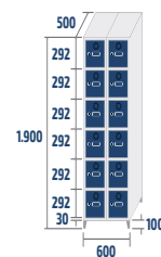
SB-30/2 COD: 43062 41,1kg · 0,57m 3
