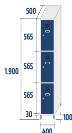
SM-40/1 COD: 44031 23,9kg · 0,38m 3
