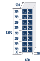
SZ-30/2 COD: 43082 45,1kg · 0,57m 3
