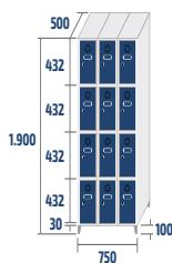
SC-25/3 COD: 42523 48,8kg · 0,71m 3
