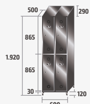
ST-30/2 INOX COD: 83912 50kg · 0,69m³
