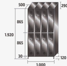
ST-25/4 INOX COD: 82914 75,1kg · 0,95m³
