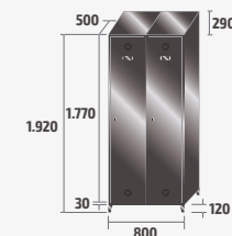
SV-40/2 INOX COD: 84902 59kg · 0,76m³
