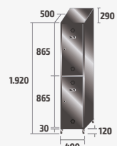
ST-40/1 INOX COD: 84911 37kg · 0,38m³
