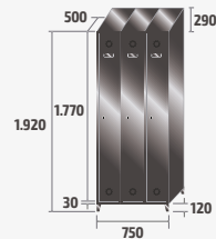
SV-25/3 INOX COD: 82903 57,8kg · 0,71m³
