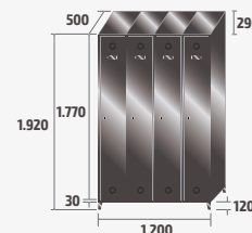
SV-30/4 INOX COD: 83904 85kg · 1,31m³
