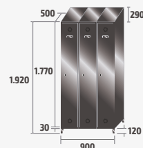
SV-30/3 INOX COD: 83903 67kg · 0,99m³
