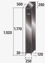
SV-25/1 INOX COD: 82901 24,6kg · 0,24m³
