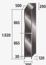
ST-30/1 INOX COD: 83911 32kg · 0,38m³
