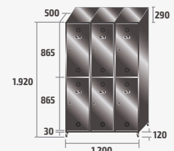
ST-40/3 INOX COD: 84913 83kg · 1,14m³
