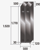
SV-25/2 INOX COD: 82902 40,3kg · 0,48m³
