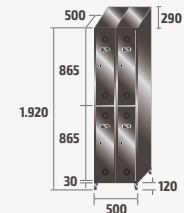
ST-25/2 INOX COD: 82912 41,3kg · 0,48m³
