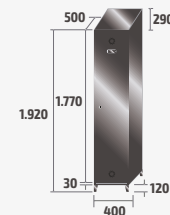
SV-40/1 INOX COD: 84901 36kg · 0,38m³
