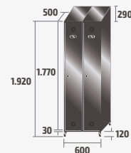
SV-30/2 INOX COD: 83902 49kg · 0,69m³
