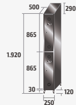
ST-25/1 INOX COD: 82911 25,6kg · 0,24m³
