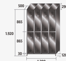
ST-30/4 INOX COD: 83914 86kg · 1,31m³
