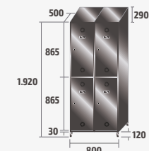
ST-40/2 INOX COD: 84912 60kg · 0,76m³
