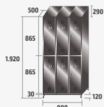
ST-30/3 INOX COD: 83913 68kg · 0,99m³
