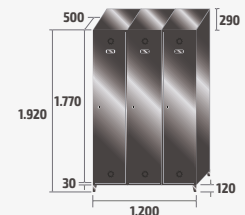
SV-40/3 INOX COD: 84903 82kg · 1,14m³
