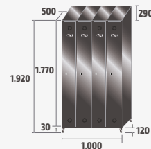
SV-25/4 INOX COD: 82904 74,1kg · 0,95m³
