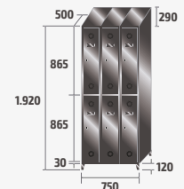
ST-25/3 INOX COD: 82913 58,8kg · 0,71m³
