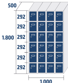
ECOB-25/4 COD: 82724 75,4kg · 0,9m 3
