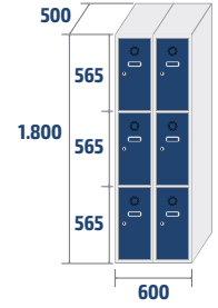
ECOM-30/2 COD: 83032 36,4kg · 0,54m 3
