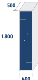
ECOL-40/1 COD: 35401 28,1kg · 0,36m 3
