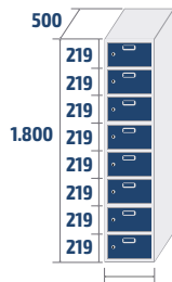
ECOZ-40/1 COD: 84821 30,9kg · 0,36m 3
