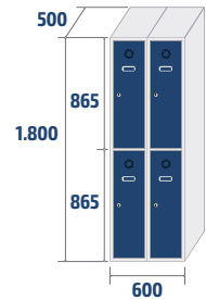
ECOT-30/2 COD: 83012 33,2kg · 0,54m 3
