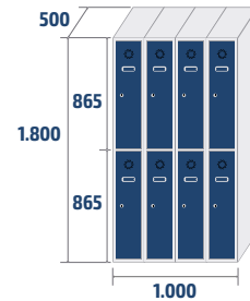
ECOT-25/4 COD: 82514 57,1kg · 0,9m 3
