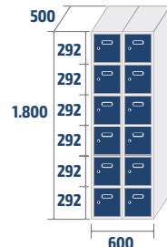
ECOB-30/2 COD: 83722 44kg · 0,54m 3
