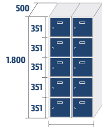
ECOP-40/2 COD: 84062 48,3kg · 0,72m 3
