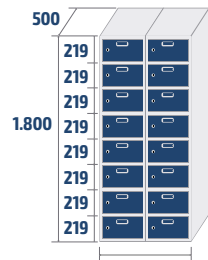
ECOZ-40/2 COD: 84822 56,8kg · 0,72m 3
