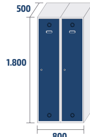
ECOV-40/2 COD: 84002 35,1kg · 0,72m 3
