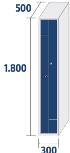
ECOL-30/1 COD: 35301 24,4kg · 0,27m 3
