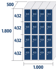
ECOC-25/4 COD: 82524 65,2kg · 0,9m 3
