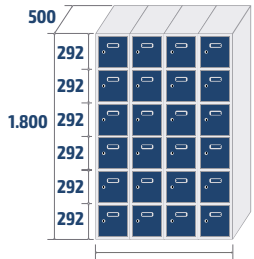
ECOB-30/4 COD: 83724 83kg · 1,08m 3
