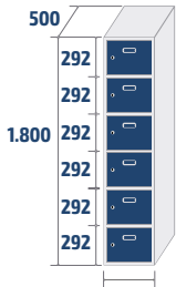
ECOB-40/1 COD: 84721 28,1kg · 0,36m 3
