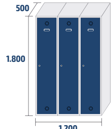
ECOV-40/3 COD: 84003 49,9kg · 1,08m 3
