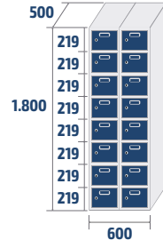
ECOZ-30/2 COD: 83822 48,4kg · 0,54m 3
