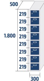
ECOZ-30/1 COD: 83821 26,7kg · 0,27m 3
