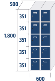
ECOP-30/2 COD: 83062 40,9kg · 0,54m 3
