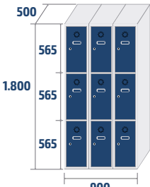
ECOM-30/3 COD: 83033 51,6kg · 0,81m 3
