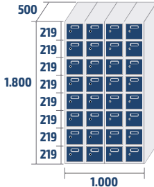
ECOZ-25/4 COD: 82584 82,6kg · 0,9m 3
