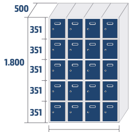
ECOP-30/4 COD: 83064 75,9kg · 1,08m 3
