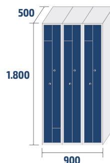
ECOL-30/3 COD: 35303 61,3kg · 0,81m 3
