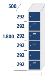
ECOB-40/1 COD: 84721 28,1kg · 0,36m 3
