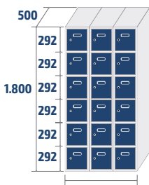
ECOB-30/3 COD: 83723 63,5kg · 0,81m 3
