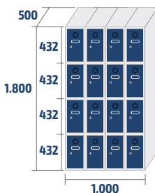
ECOC-25/4 COD: 82524 65,2kg · 0,9m 3
