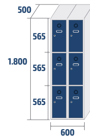
ECOM-30/2 COD: 83032 36,4kg · 0,54m 3
