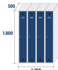
ECOV-30/4 COD: 83004 59,5kg · 1,08m 3
