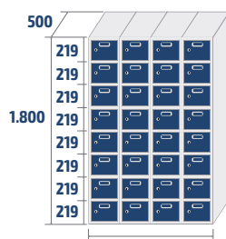
ECOZ-30/4 COD: 83824 91,8kg · 1,08m 3
