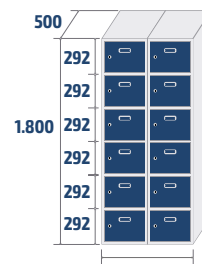
ECOB-40/2 COD: 84722 51,2kg · 0,72m 3
