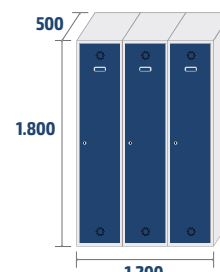
ECOV-40/3 COD: 84003 49,9kg · 1,08m 3
