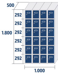
ECOB-25/4 COD: 82724 75,4kg · 0,9m 3
