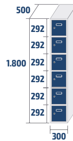
ECOB-30/1 COD: 83721 24,5kg · 0,27m 3
