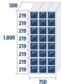
ECOZ-25/3 COD: 82583 63,2kg · 0,67m 3
