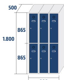
ECOT-30/3 COD: 83013 47,3kg · 0,81m 3
