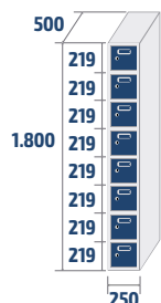
ECOZ-25/1 COD: 82581 24,4kg · 0,22m 3
