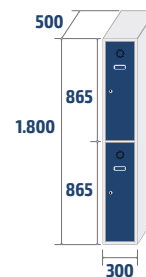
ECOT-30/1 COD: 83011 19,1kg · 0,27m 3
