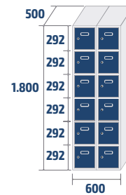
ECOB-30/2 COD: 83722 44kg · 0,54m 3
