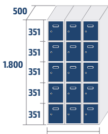
ECOP-30/3 COD: 83063 58,4kg · 0,81m 3
