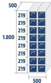
ECOZ-25/2 COD: 82582 43,8kg · 0,45m 3
