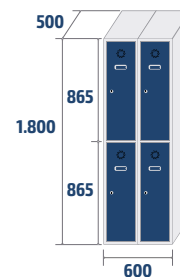
ECOT-30/2 COD: 83012 33,2kg · 0,54m 3
