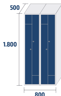
ECOL-40/2 COD: 35402 50,2kg · 0,72m 3
