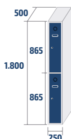
ECOT-25/1 COD: 82511 18,4kg · 0,22m 3
