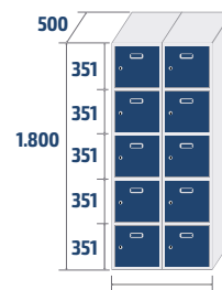
ECOP-40/2 COD: 84062 48,3kg · 0,72m 3
