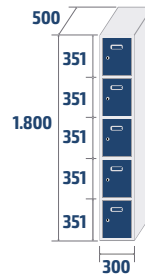
ECOP-30/1 COD: 83621 23,4kg · 0,27m 3
