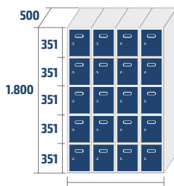
ECOP-30/4 COD: 83064 75,9kg · 1,08m 3
