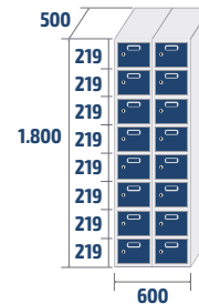
ECOZ-30/2 COD: 83822 48,4kg · 0,54m 3
