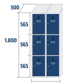
ECOM-40/2 COD: 84032 42,4kg · 0,72m 3
