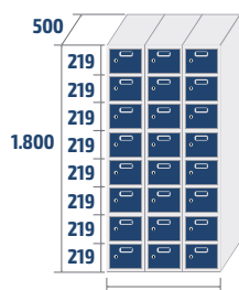
ECOZ-30/3 COD: 83823 70,1kg · 0,81m 3
