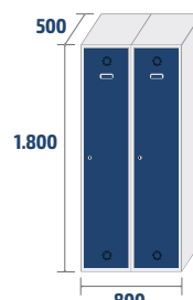
ECOV-40/2 COD: 84002 35,1kg · 0,72m 3
