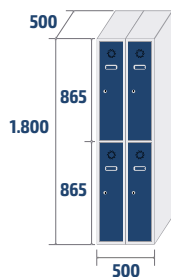
ECOT-25/2 COD: 82512 31,3kg · 0,45m 3
