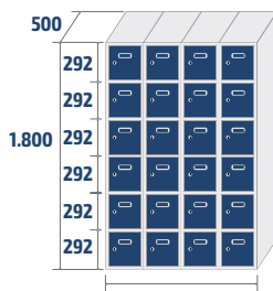
ECOB-30/4 COD: 83724 83kg · 1,08m 3
