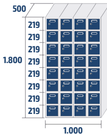
ECOZ-25/4 COD: 82584 82,6kg · 0,9m 3
