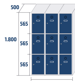
ECOM-40/3 COD: 84033 60,6kg · 1,08m 3
