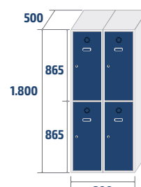
ECOT-40/2 COD: 84012 41kg · 0,72m 3
