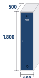
ECOV-40/1 COD: 84001 20,3kg · 0,36m 3
