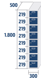
ECOZ-30/1 COD: 83821 26,7kg · 0,27m 3
