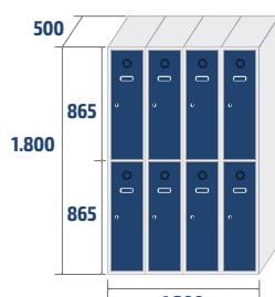
ECOT-30/4 COD: 83014 61,4kg · 1,08m 3
