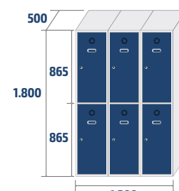
ECOT-40/3 COD: 84013 59kg · 1,08m 3
