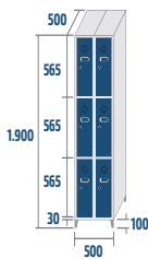
SM-25/2 COD: 42532 33,2kg · 0,48m 3
