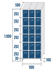
SB-30/3 COD: 43063 59,1kg · 0,86m 3
