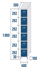
SB-40/1 COD: 44061 27kg · 0,38m 3
