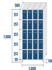
SP-25/4 COD: 42554 67,4kg · 0,95m 3
