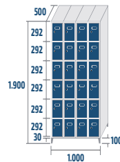
SB-25/4 COD: 42564 71,4kg · 0,95m 3
