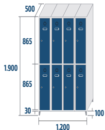
ST-30/4 COD: 43014 62,2kg · 1,14m 3
