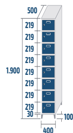
SZ-40/1 COD: 44081 29kg · 0,38m 3
