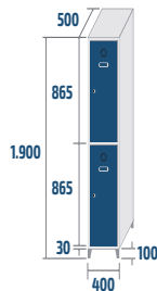
ST-40/1 COD: 44011 23kg · 0,38m 3
