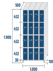
SC-25/4 COD: 42524 63,4kg · 0,95m 3
