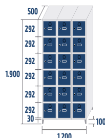
SB-40/3 COD: 44063 69kg · 1,14m 3
