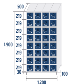
SZ-30/4 COD: 43084 85,2kg · 1,14m 3
