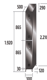
ST-30/1 INOX COD: 83911 31kg · 0,38m 3
