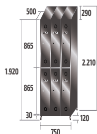
ST-25/3 INOX COD: 82913 57,8kg · 0,71m 3
