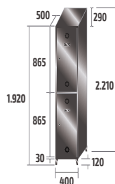
ST-40/1 INOX COD: 84911 36kg · 0,38m 3
