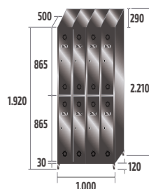
ST-25/4 INOX COD: 82914 74,1kg · 0,95m 3
