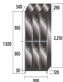
ST-30/3 INOX COD: 83913 67kg · 0,99m 3
