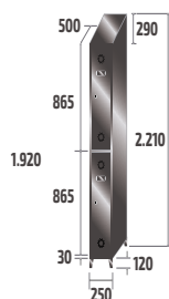
ST-25/1 INOX COD: 82911 24,6kg · 0,24m 3
