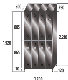
ST-30/4 INOX COD: 83914 85kg · 1,31m 3
