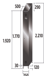
SV-25/1 INOX COD: 82901 24,6kg · 0,24m 3
