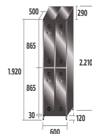
ST-30/2 INOX COD: 83912 49kg · 0,69m 3
