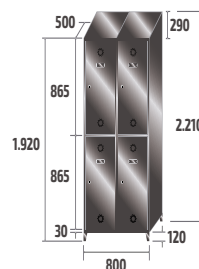
ST-40/2 INOX COD: 84912 59kg · 0,76m 3
