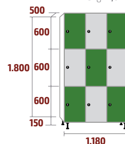
FM-40/3 COD: 53135 133kg · 1,06m 3
