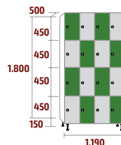
FC-30/4 COD: 53143 158kg · 1,07m 3
