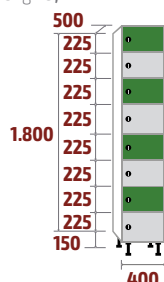
FZ-40/1 COD: 53082 70kg · 0,36m 3
