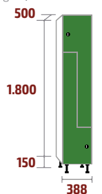
FL-40/1 COD: 53042 56kg · 0,36m 3
