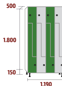
FL-30/4 COD: 53183 175kg · 1,07m 3
