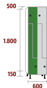
FL-30/2 COD: 53181 92kg · 0,54m 3
