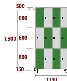
FM-30/4 COD: 53133 148kg · 1,07m 3
