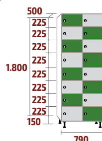
FZ-40/2 COD: 53174 127kg · 0,71m 3
