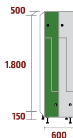
FL-30/2 COD: 53181 92kg · 0,54m 3
