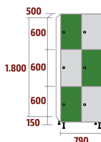
FM-40/2 COD: 53134 93kg · 0,71m 3
