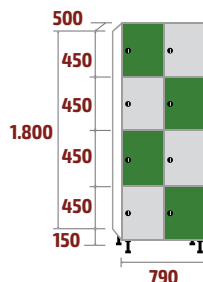
FC-40/2 COD: 53144 99kg · 0,71m 3
