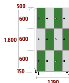
FM-30/4 COD: 53133 148kg · 1,07m 3
