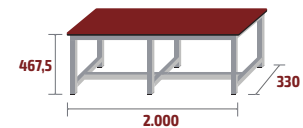
BANC-1-2000-FEN COD: 79503 · 24kg · 0,33m 3
