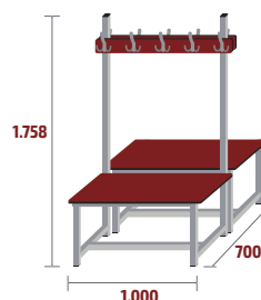
BANC-2-1000-FEN-DC COD: 79554 · 48kg · 0,46m 3 · 10 ↓
