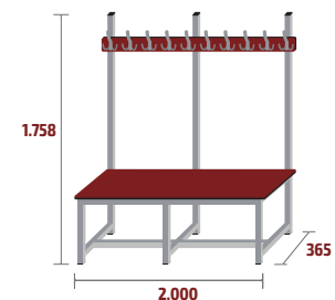
BANC-2-2000-FEN COD: 79506 · 37kg · 0,31m 3 · 10 ↓
