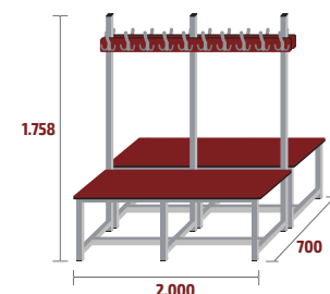
BANC-2-2000-FEN-DC COD: 79556 · 74kg · 0,62m 3 · 20 ↓
