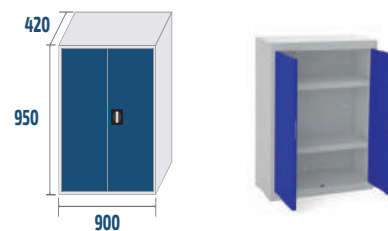
ARM05 COD: 90001 2 bandejas grandes
