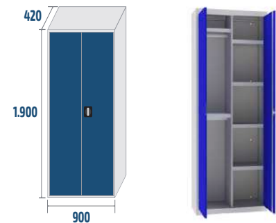
ARM06 COD: 19006 Separador grande + 6 medias bandejas + 2 barras colgador
