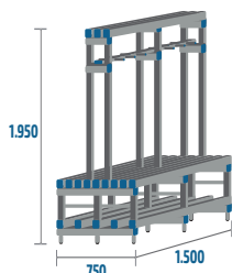
BANC-3-PVC-1500-DC COD: 79164 · 39kg · 0,75m 3 · 12 ↓
