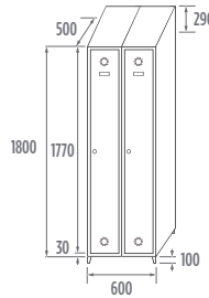
SV-30/2 INOX COD. 83902
