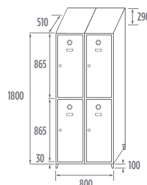
ST-40/2 INOX COD. 84912
