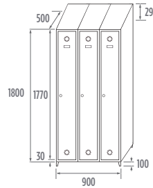
SV-30/3 INOX COD. 83903
