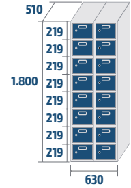
AZ-30/2 COD: 33082 49,5kg · 0,58m 3
