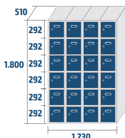
AB-30/4 COD: 33064 84,2kg · 1,13m 3
