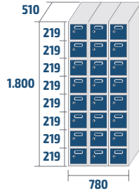
AZ-25/3 COD: 32583 64,2kg · 0,72m 3
