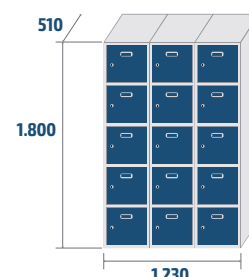
AP-40/3 COD: 34053 72,3kg · 1,13m 3
