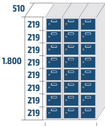
AZ-30/3 COD: 33083 71,2kg · 0,85m 3
