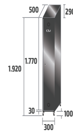
SV-30/1 INOX COD: 83901 31kg · 0,38m 3
