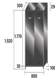
SV-40/2 INOX COD: 84902 59kg · 0,76m 3
