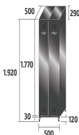
SV-25/2 INOX COD: 82902 40,3kg · 0,48m 3
