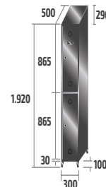
SV-30/1 INOX COD: 83901 31kg · 0,38m 3
