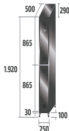
SV-25/1 INOX COD: 82901 24,6kg · 0,24m 3
