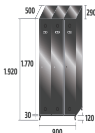
SV-30/3 INOX COD: 83903 67kg · 0,99m 3
