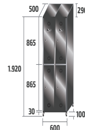
SV-30/2 INOX COD: 83902 49kg · 0,69m 3
