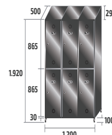
SV-40/3 INOX COD: 84903 82kg · 1,14m 3
