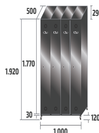
SV-25/4 INOX COD: 82904 74,1kg · 0,95m 3
