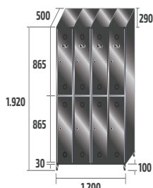
SV-30/4 INOX COD: 83904 85kg · 1,31m 3
