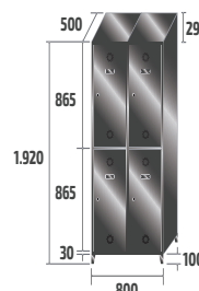
SV-40/2 INOX COD: 84902 59kg · 0,76m 3
