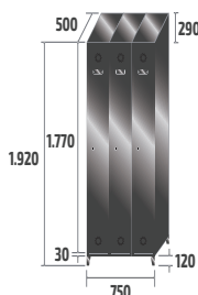
SV-25/3 INOX COD: 82903 57,8kg · 0,71m 3
