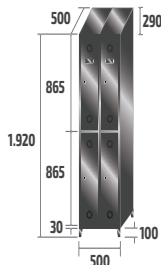
SV-25/2 INOX COD: 82902 40,3kg · 0,48m 3
