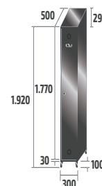
SV-30/1 INOX COD: 83901 31kg · 0,38m 3
