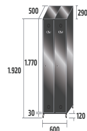
SV-30/2 INOX COD: 83902 49kg · 0,69m 3
