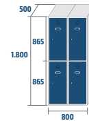
ST-40/2-PLUS
