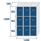
SM-40/3-PLUS
