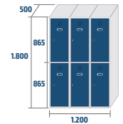
ST-40/3-PLUS
