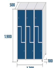
SL2-40/3 COD: 43145 63kg · 1,14m 3
