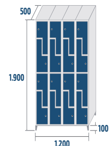
SL4-30/4 COD: 43153 69,1kg · 1,14m 3
