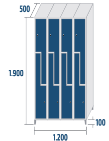
SL2-30/4 COD: 43143 69,1kg · 1,14m 3
