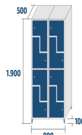
SL4-40/2 COD: 43055 44kg · 0,76m 3
