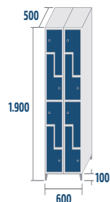
SL4-30/2 COD: 43052 37,1kg · 0,57m 3
