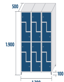
SL4-40/3 COD: 43155 63kg · 1,14m 3
