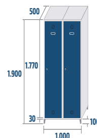
SV-50/2 COD: 45002 51kg · 0,95m 3
