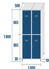
ST-50/2 COD: 45012 47kg · 0,95m 3
