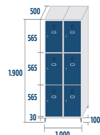
SM-50/2 COD: 45032 46,6kg · 0,95m 3
