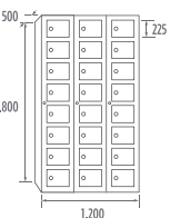
STV8-40/3 COD. 44083
