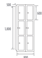
STV3-40/2 COD. 44032
