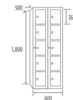
STV5-40/2 COD. 44052
