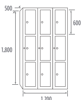
STV3-40/3 COD. 44033
