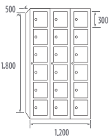
STV6-40/3 COD. 44063
