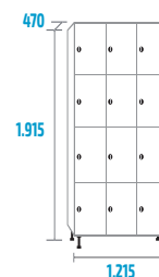
PC-40/3 COD: 22038
